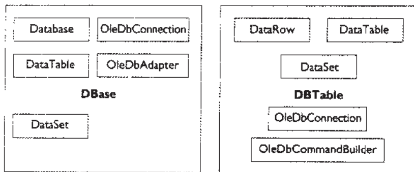
图 18.2 Facade 将类包装，组成了 DBase 类和 DBTable 类
