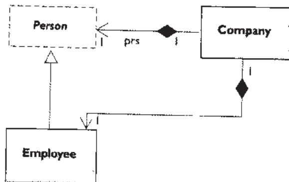
图 6.5 Company 类包含了 Person 和 Employee 实例
