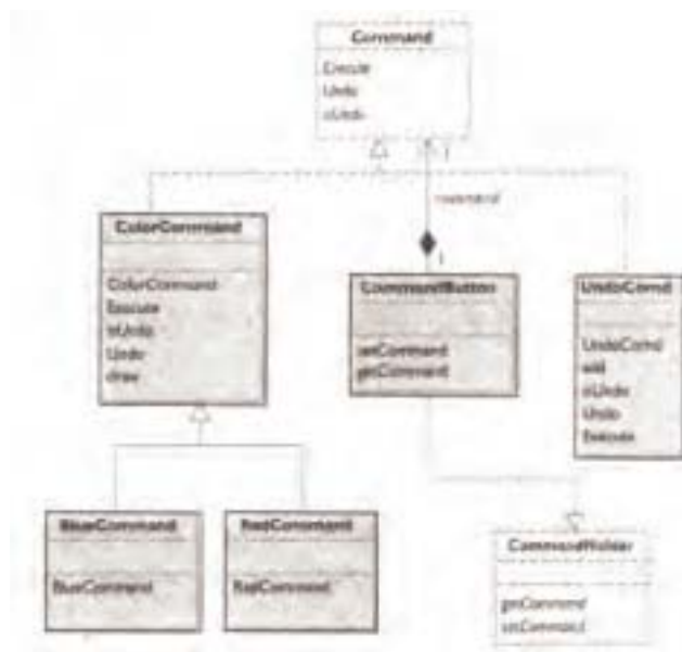
图 22.7 在命令模式中实现 Undo 操作的类图
