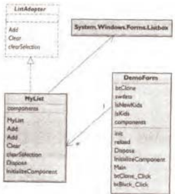
图 14.4 列表适配器的类适配器方法
