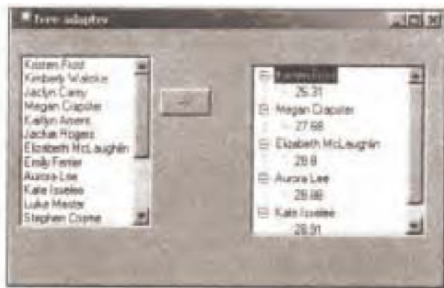
图 14.3 TreeDemo 程序
