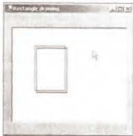
图 5.5 DoubleRect 类
