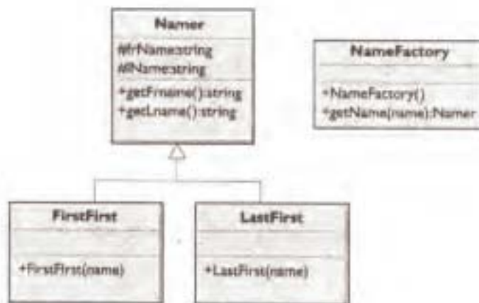
图 8.2 NameFactory 程序
